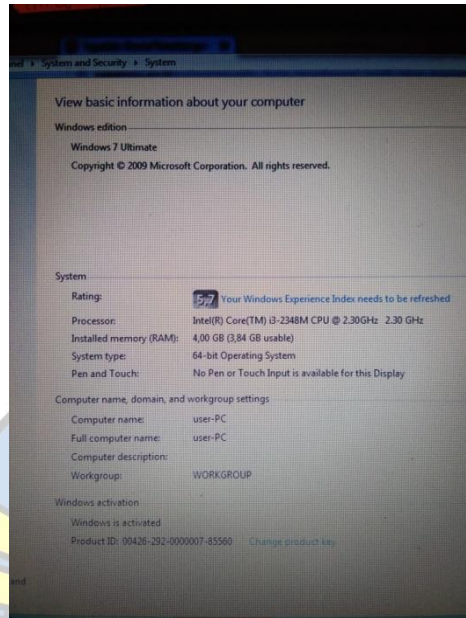
Gambar 3.5 Spesifikasi Laptop
