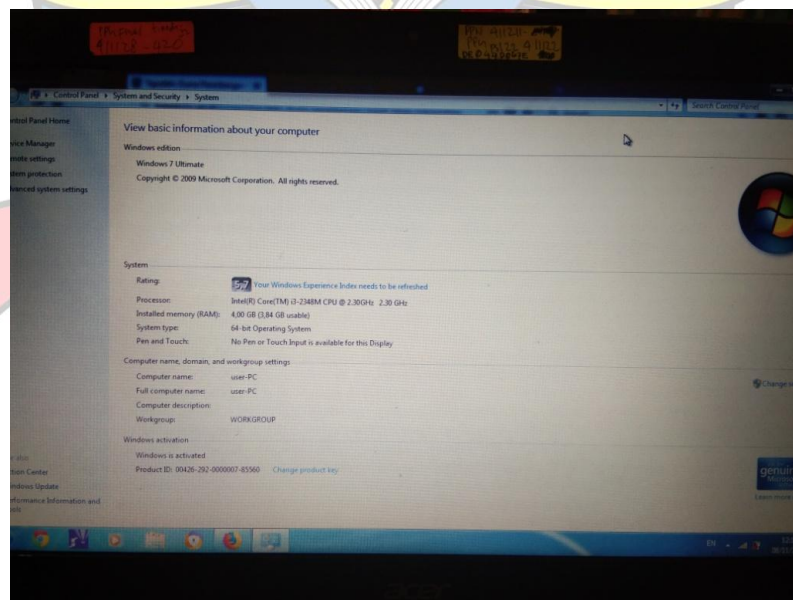
Gambar 3.4 Spesifikasi Laptop
