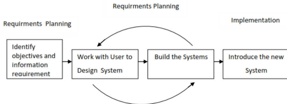
Gambar 1.1. Metode RAD [6]
