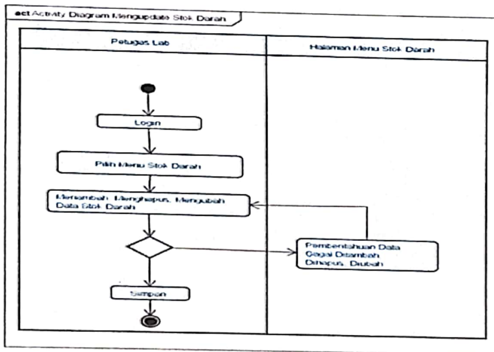
Gambar 5.4 Activity Diagram Mengupdate Stok Darah
