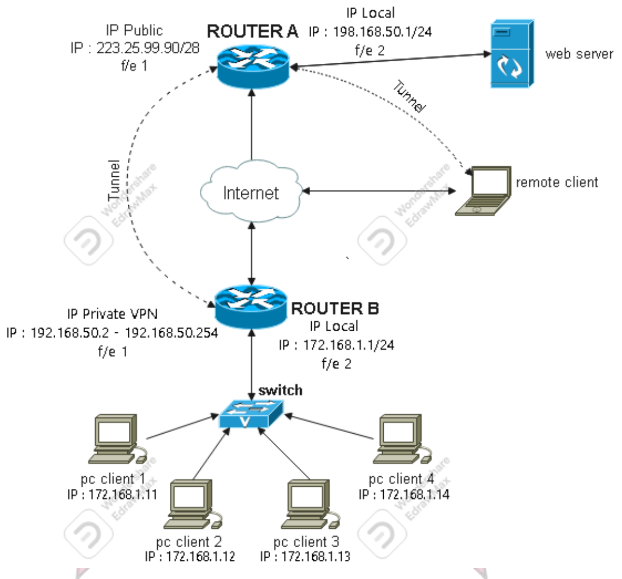
Gambar 4.3. Rancangan Topologi
